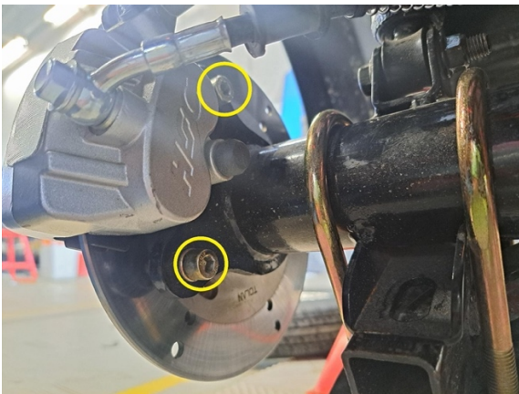
Irrota takajarrusatulan kiinnityspulttit. (kuusiokoloavain 6 mm).
